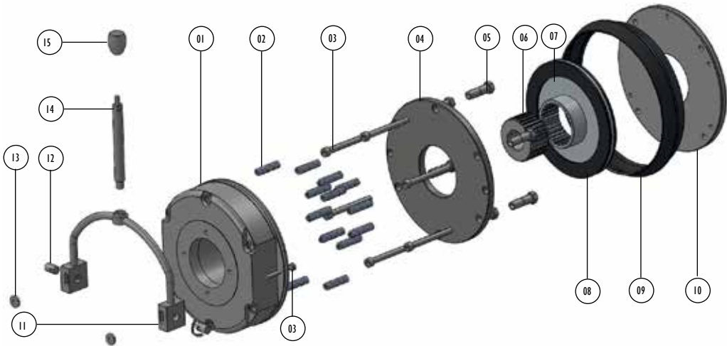
3D Explosionszeichnung ERB
