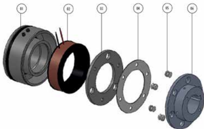
3D Explosionszeichnung Typ 101
