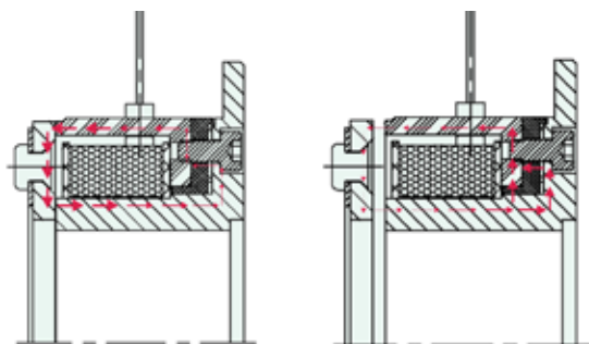
Bremse aktiviert
