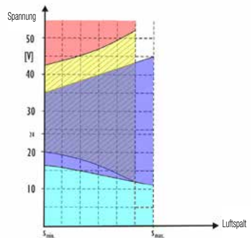
Freigabe Diagramm der Bremse
