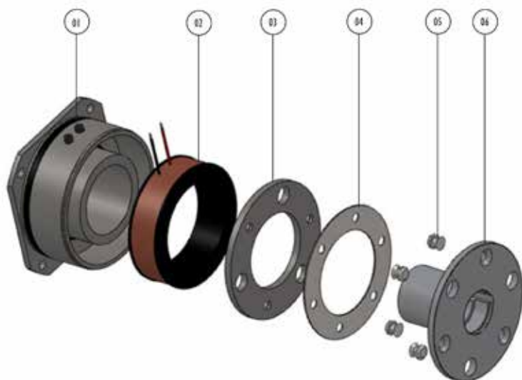
3D Explosionszeichnung Typ 102
